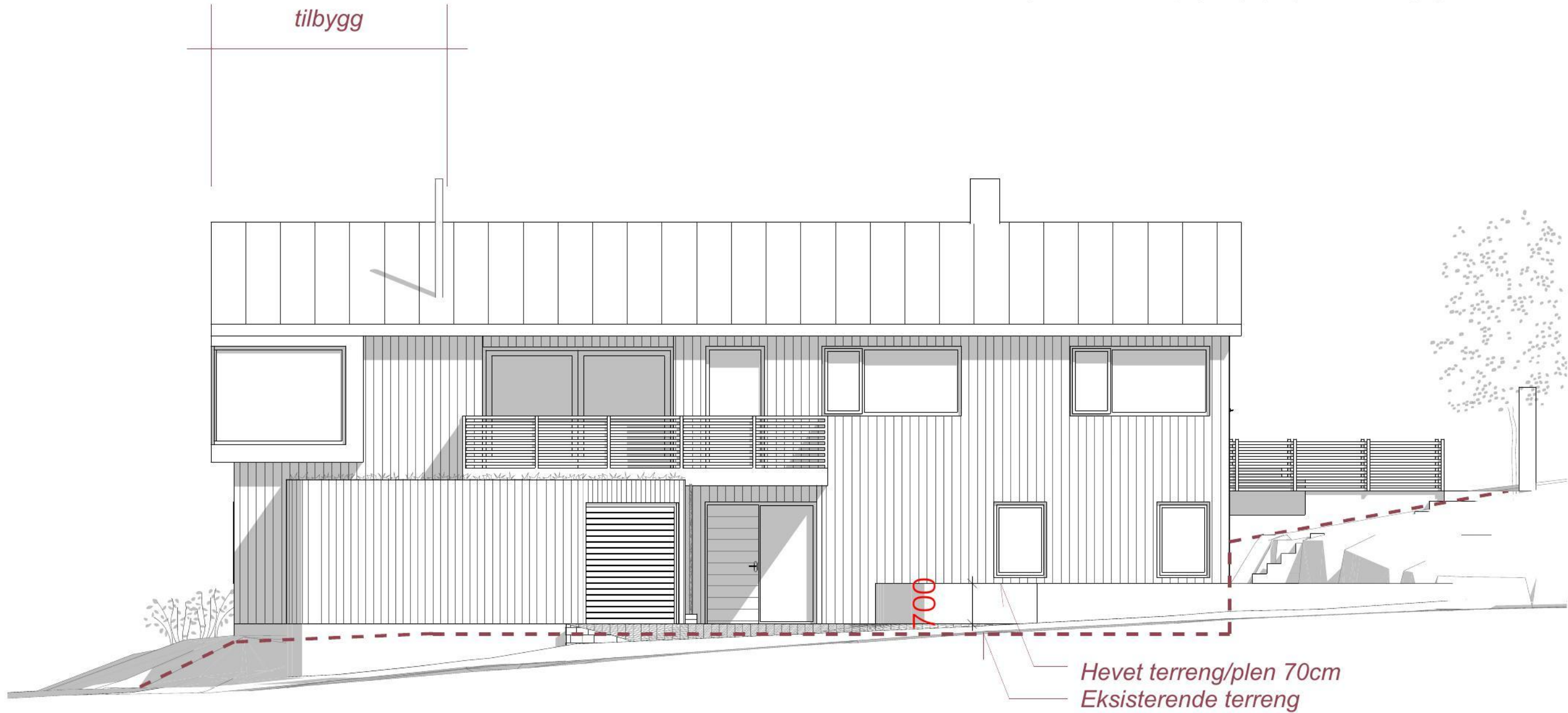
1:100 Fasade Vest
